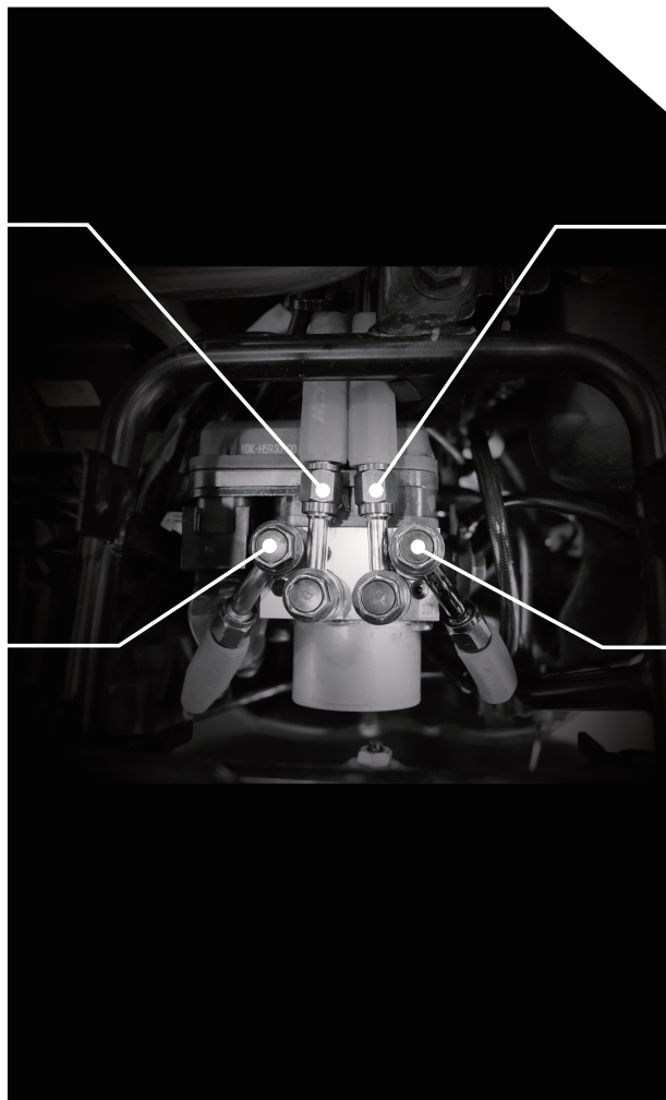
(95cm, 1彎1直) 彎頭在ABS電腦端 另一直頭連接 前卡鉗 95cm: straight-> front caliper bent-> ABS
