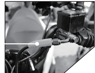
(45cm-1彎1直) 直頭在ABS電腦端 另一彎頭連接 左拉桿 45cm: bent-> left lever straight-> ABS
