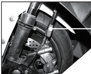
(95cm, 1彎1直) 彎頭在ABS電腦端 另一直頭連接 前卡鉗 95cm: straight-> front caliper bent-> ABS
