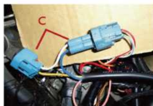
3.將線組C的DCP接頭公母插接上，(藍線須對藍線)
