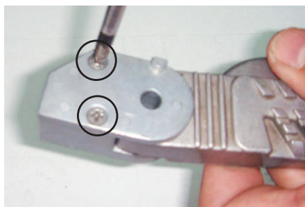
1.原車腳踏桿螺絲拆下。 Remove screws of original footrest rod set.
